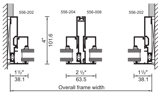
1 JAMB
